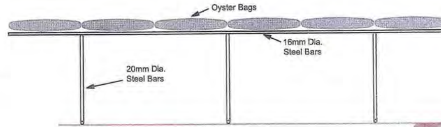
Longitudinal Section
